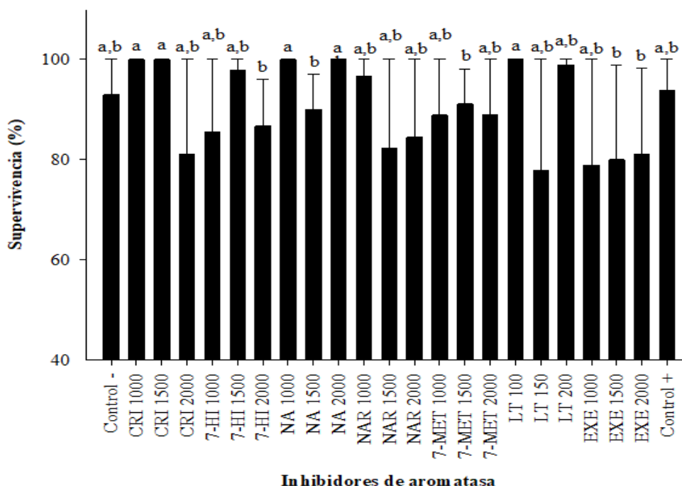
Figura 2. Promedio \pm desviación estándar de la supervivencia (%) de crías de O. niloticus , tratadas con diferentes inhibidores de la aromatasa. CRI: crisina, 7-HI: 7-hidroxiflavona, NA: apigenina, NAR: naringenina, 7-MET: 7-metoxiflavona, EXE: exemestano incluidas a 1000, 1500 y 2000 mg kg -1 de alimento, LT: letrozol incluido a 100, 150 y 200 mg kg -1 de alimento, Control +: 17- \alpha -metiltestosterona incluido a 60 mg kg -1 de alimento. Letras distintas en las columnas representan diferencias significativas ( P < 0.05 ).
