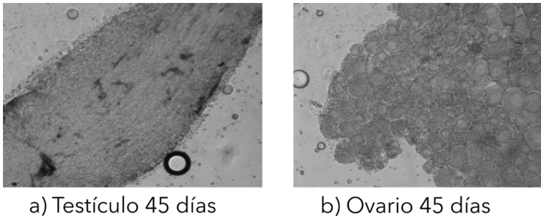
Figura 1. Visualización de las muestras de gónadas de los organismos experimentales para determinación de las proporciones de machos y hembras por tratamiento (1 a 1.5 g peso promedio individual, 2 a 3 cm longitud total), post 45 días de inicio de la alimentación con los tratamientos de andrógenos e inhibidores naturales y sintéticos de la aromatasa. Lado derecho: izquierdo, lado derecho ovario con folículos claramente visibles.
